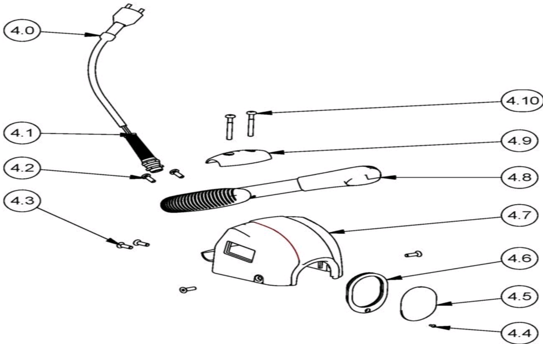
Bona Edge AM0003135 Edge machine cap
