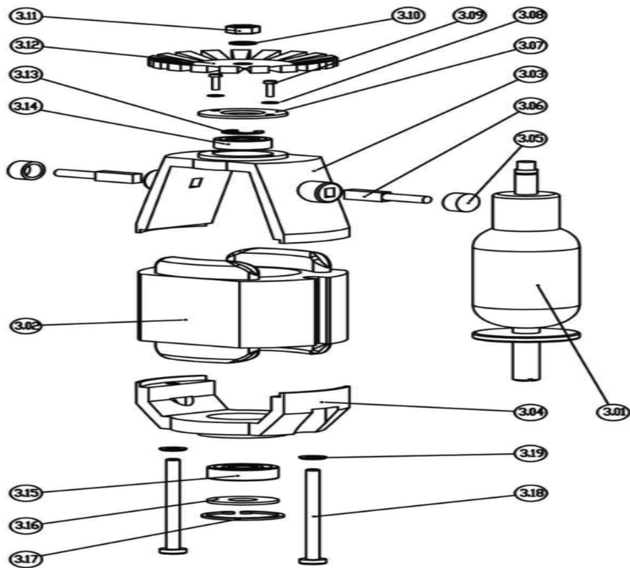
Bona Mini Edge AMO260004.0 Mini Edge Motor 115V
