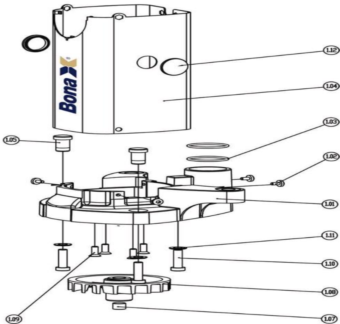
Bona Mini Edge AMO260004.0 Mini Edge Motor Bracket
