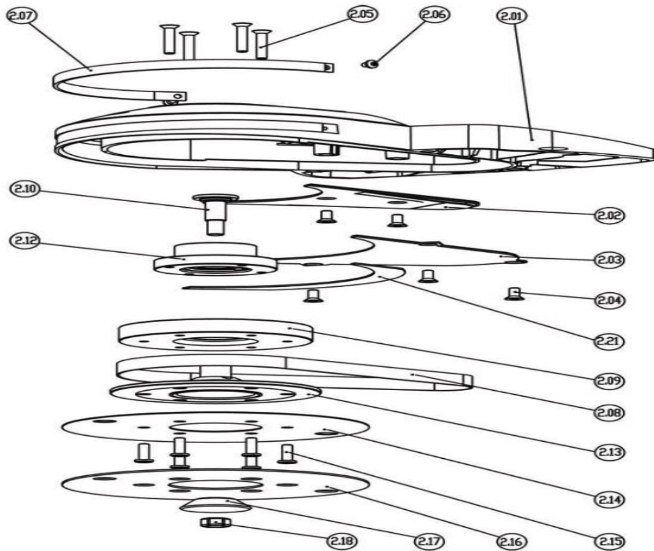
Bona Mini Edge AMO260004.0 Mini Edge sanding arm standard
