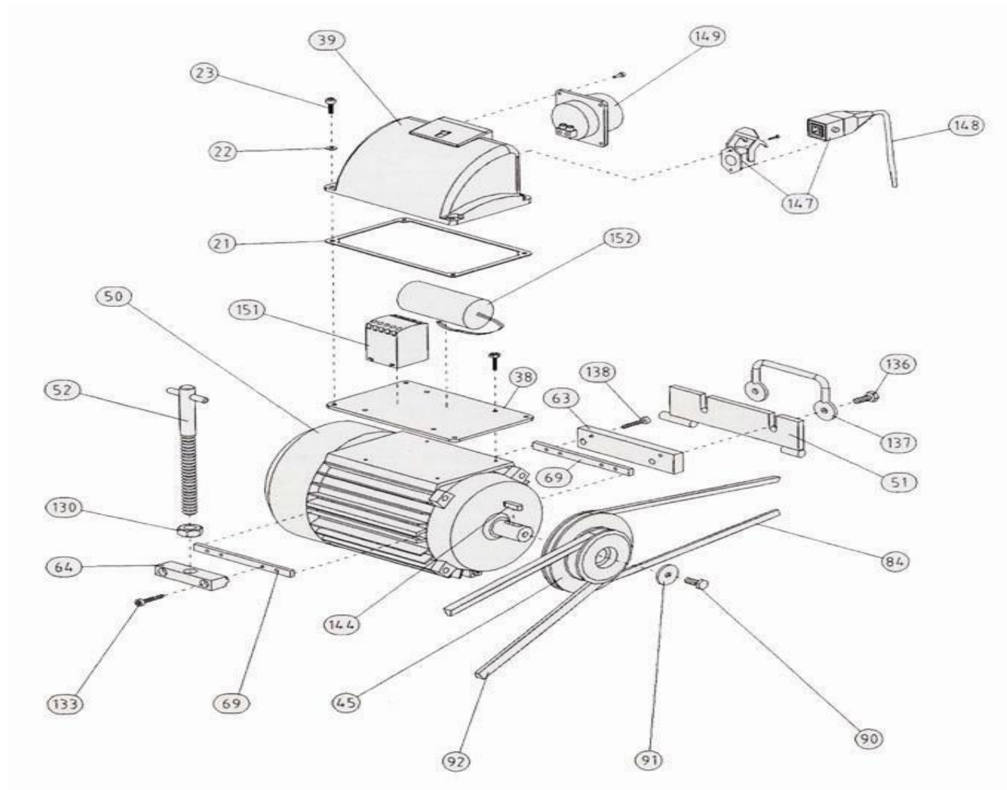
Bona Midi AMO150003.0 Midi Motor 2,2KW
