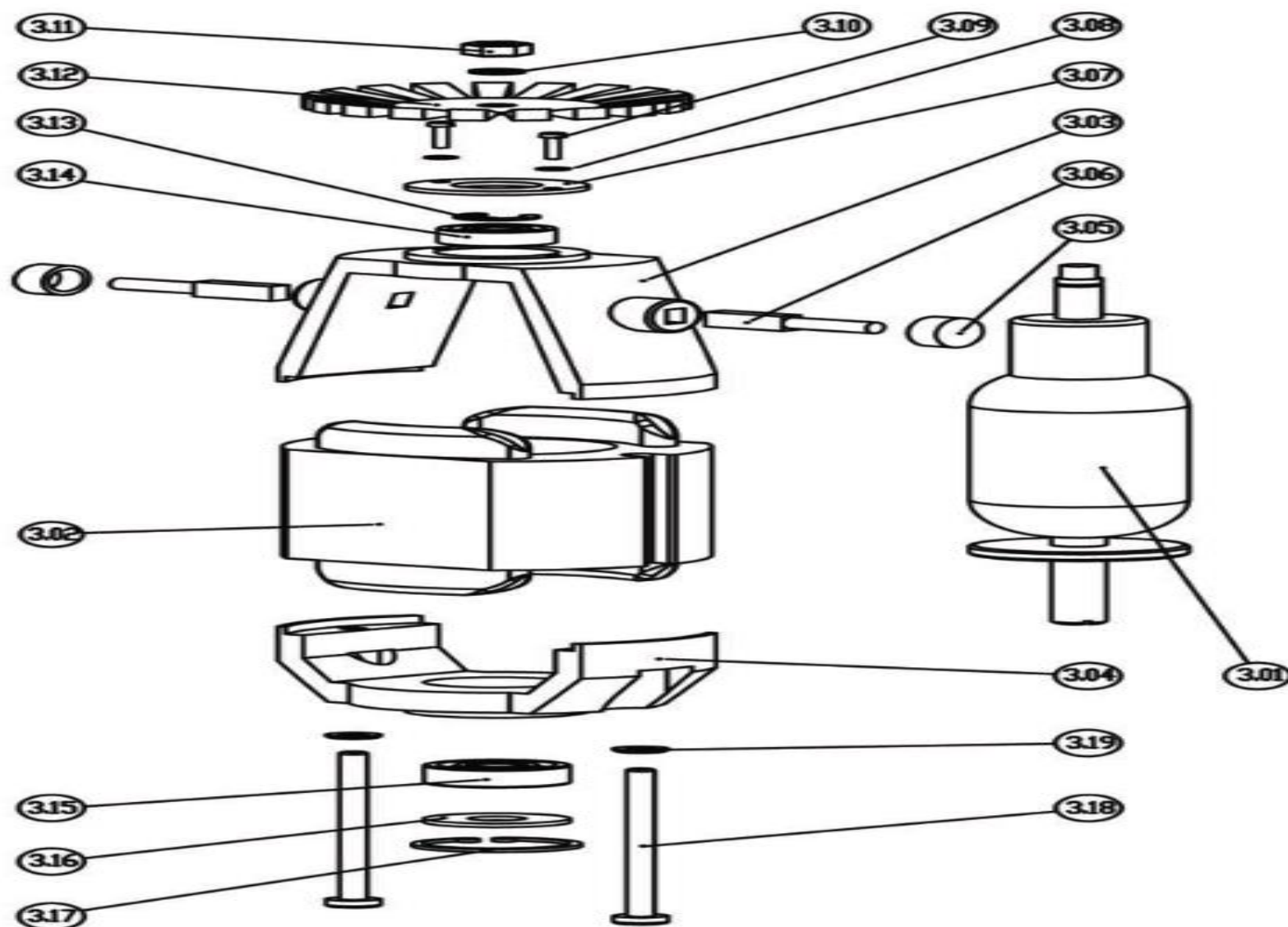
Bona Mini Edge AM0003148 Mini Edge Motor 115V
