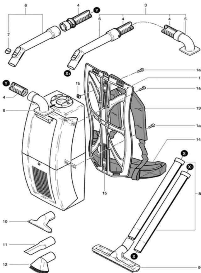
RS 05 Rückentragteil und Saugset / Pièce à porter du dos cpl. / Back carrying frame cpl. B 4-03.2002
