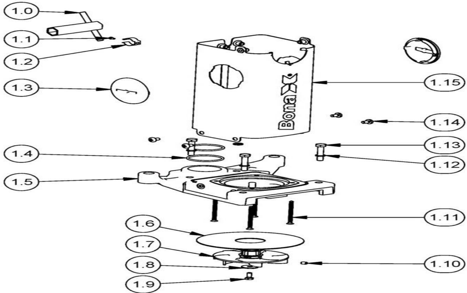
Bona Edge AMO230010.3 Edge housing
